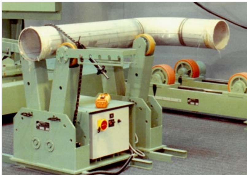
R025 con KIT T per rotazione tubi inox, con catena speciale con rulli rivestiti in Nylon
